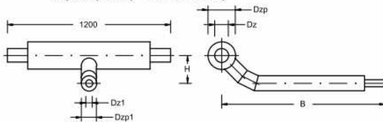
Trójnik opadowy - odwodnieniowy
